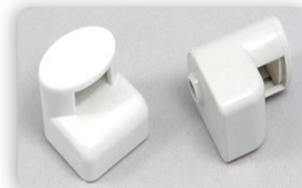
SI5M GLASS TAG RF geeignet für: Brillen, Sonnenbrillen Dimensionen für Brillengestell: 12x6.4 mm Dimensionen: 25x23x27 mm *
